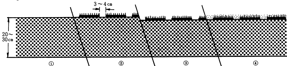
図 芝の張り方
